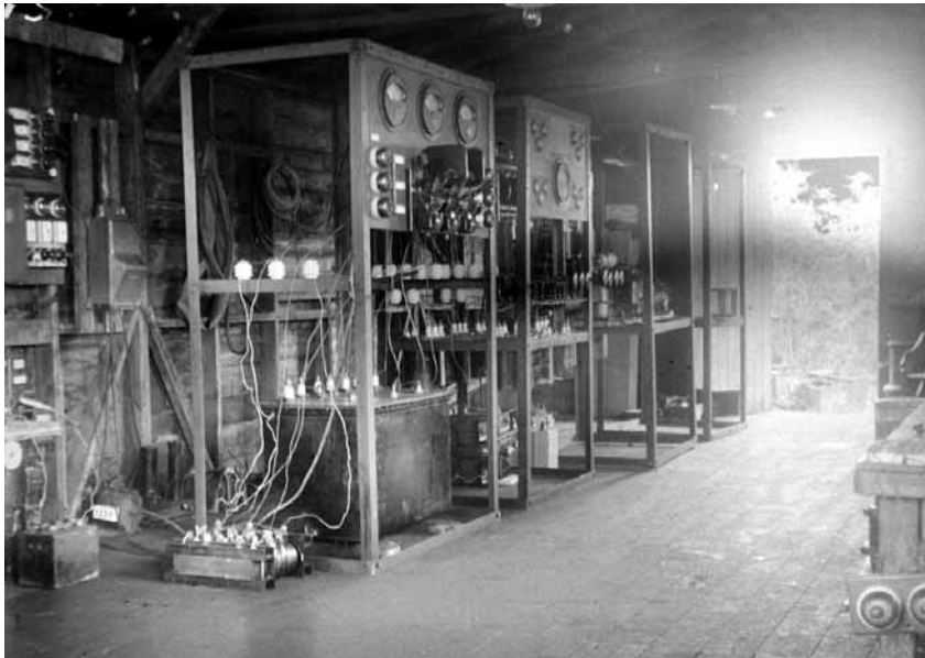
Útsendingarstöðin fyrir trúboðaútlarp Gooks uppsett. (Mynd: Minjasafnið á Akureyri)
