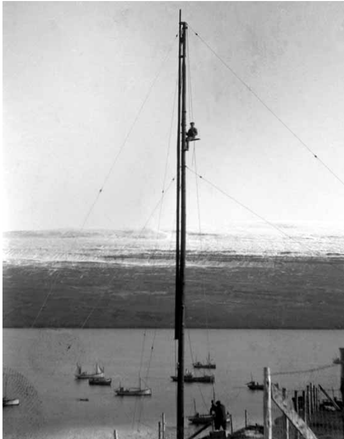
Loftnetsmöstrin sett upp – þau voru tvö 110 og 114 feta (um 35 m) há. (Mynd: Minjasafnið á Akureyri)
