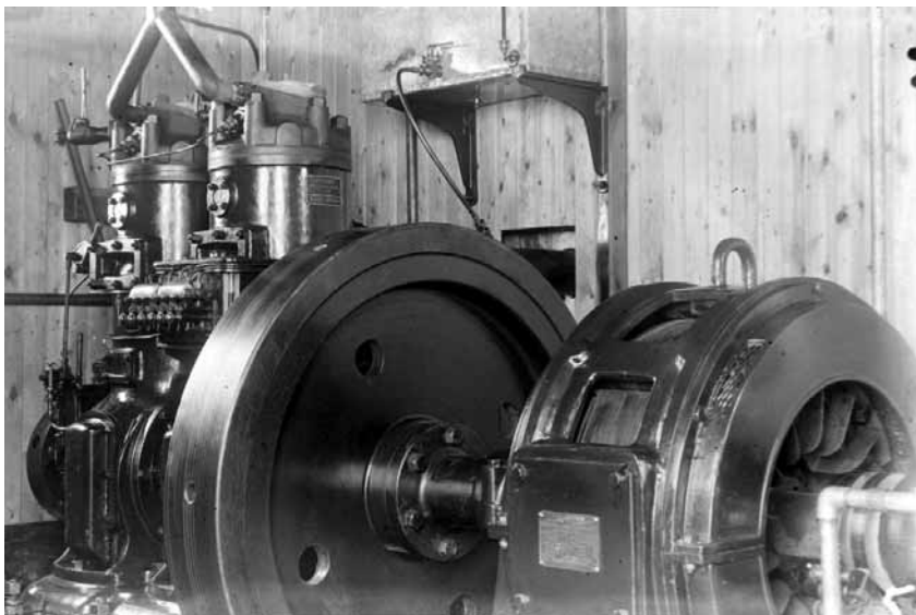
Nýja rafstöðin. (Mynd: Minjasafnið á Akureyri)
